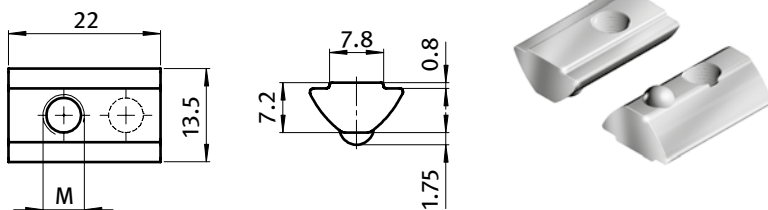
Roll-in T-slot Nut 13.5 x 7.2 mm with Spring Loaded Ball Nutenstein 13,5 x 7,2 mm, einschwenkbar mit Federkugel
