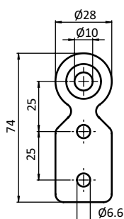
T-connector Plate D28 T-Verbinderplatte D28
