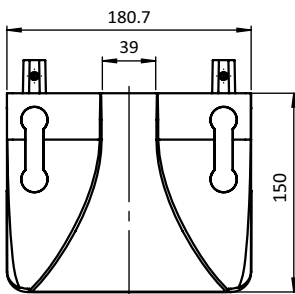
Infeed Cap for Guiding Rail FIFO (Set) Einführungskappe für Führungsschiene FIFO (Set)
